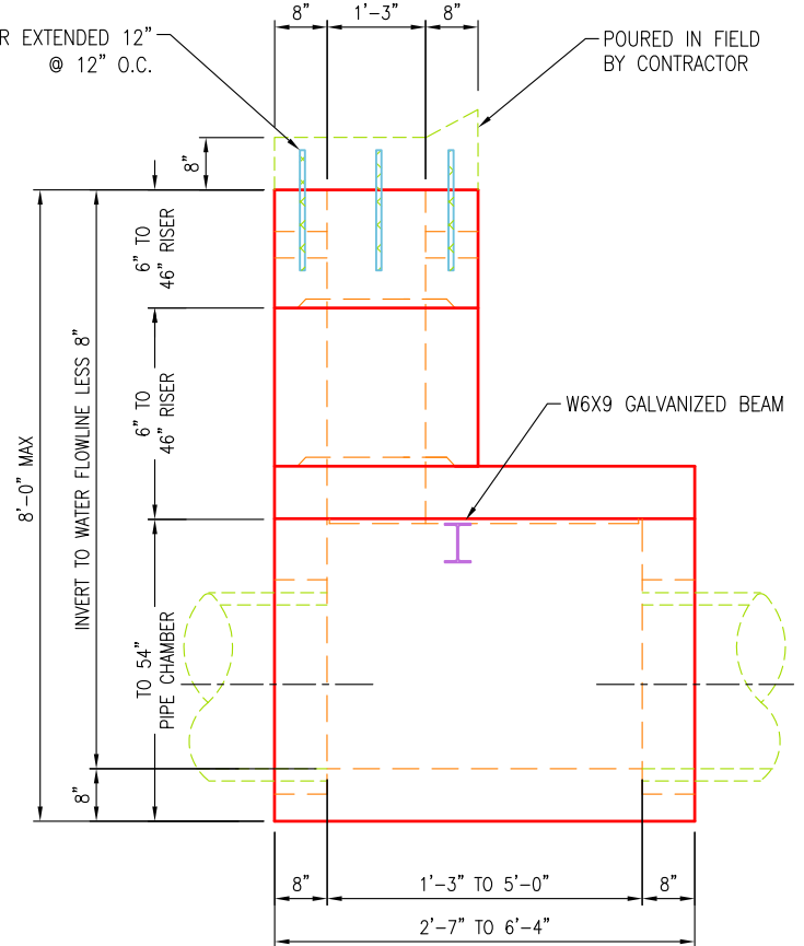
SECTION A-A
